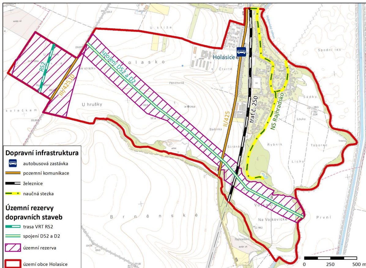
Obr. 16 Dopravní infrastruktura obce Holasice v roce 2016, včetně územních rezerv dopravních staveb.
